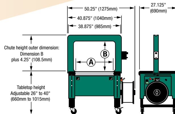
HBX-4300 Chute inner dimensions
